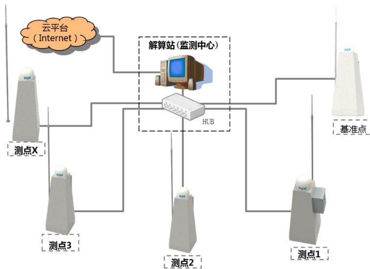
2-1 系统组成示意图
