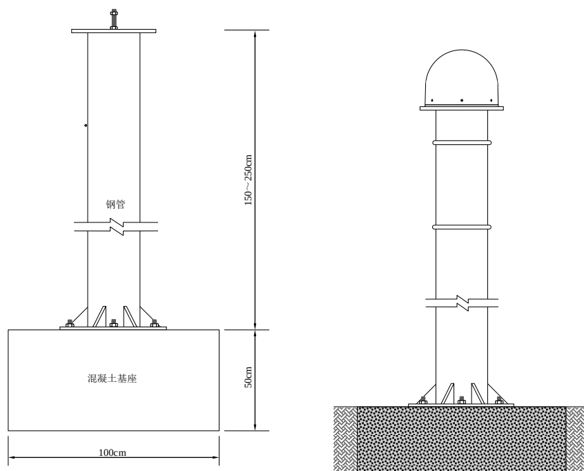
图 3-2 支架安装示意图
