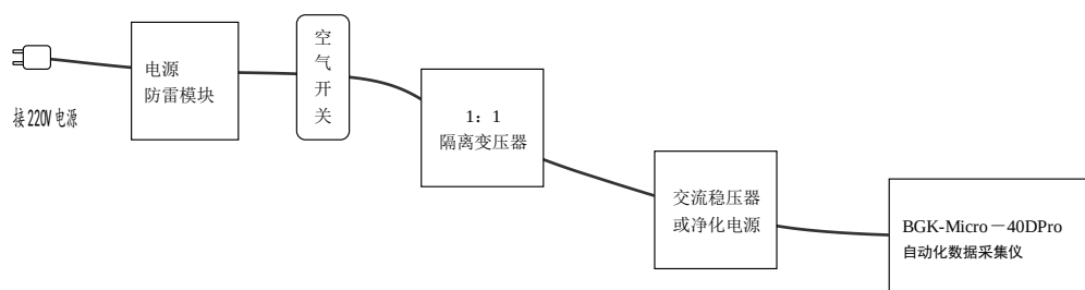
图 4.6 电源防雷连接示意图
