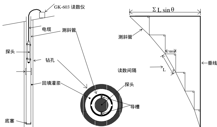
图 1.1.3 测斜仪观测图解
