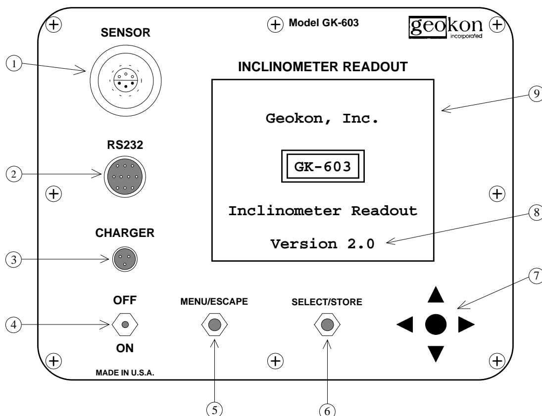
图 1.2-1 GK-603 面板
