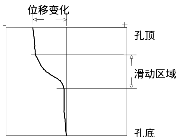
图 1.1-4 钻孔位移曲线
