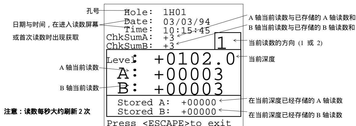
图 3.1-9 读数屏幕
